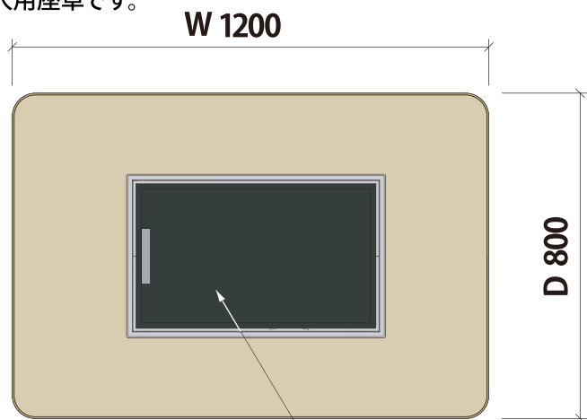
調理鉄板(590×344)
