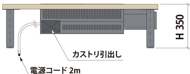
調理鉄板(590×344)
